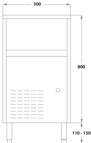
Frontansicht
