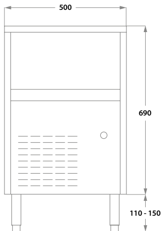
Frontansicht
