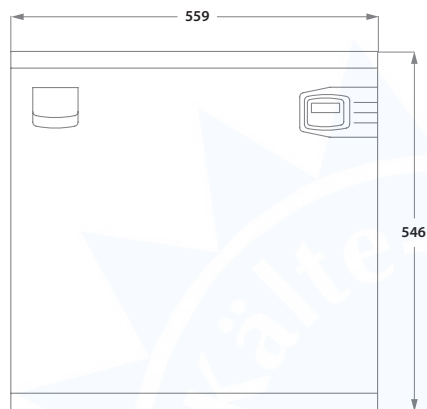
Frontansicht
