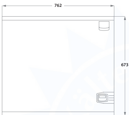
Frontansicht
