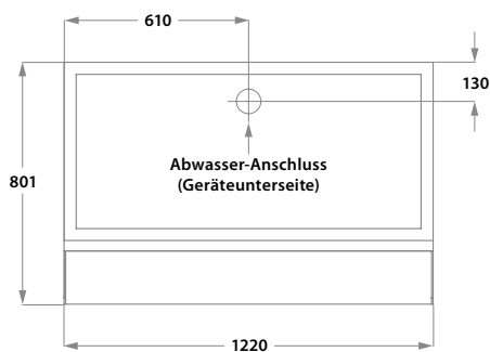
Draufsicht
