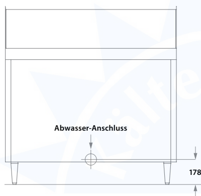
Rückansicht
