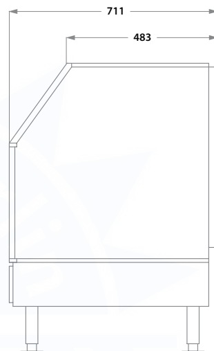
Seitenansicht
