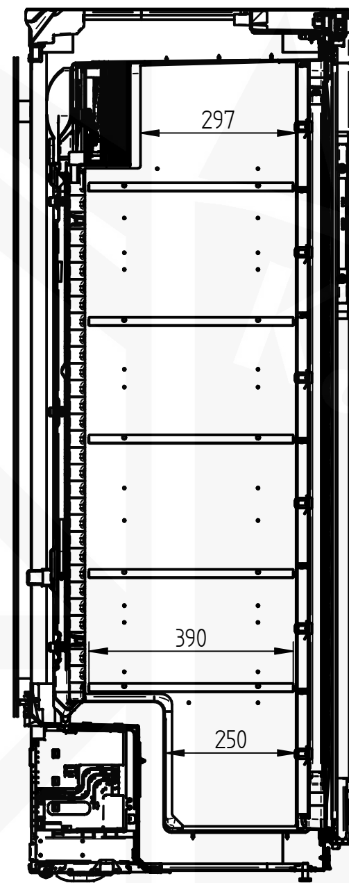
Schnitt A-A
