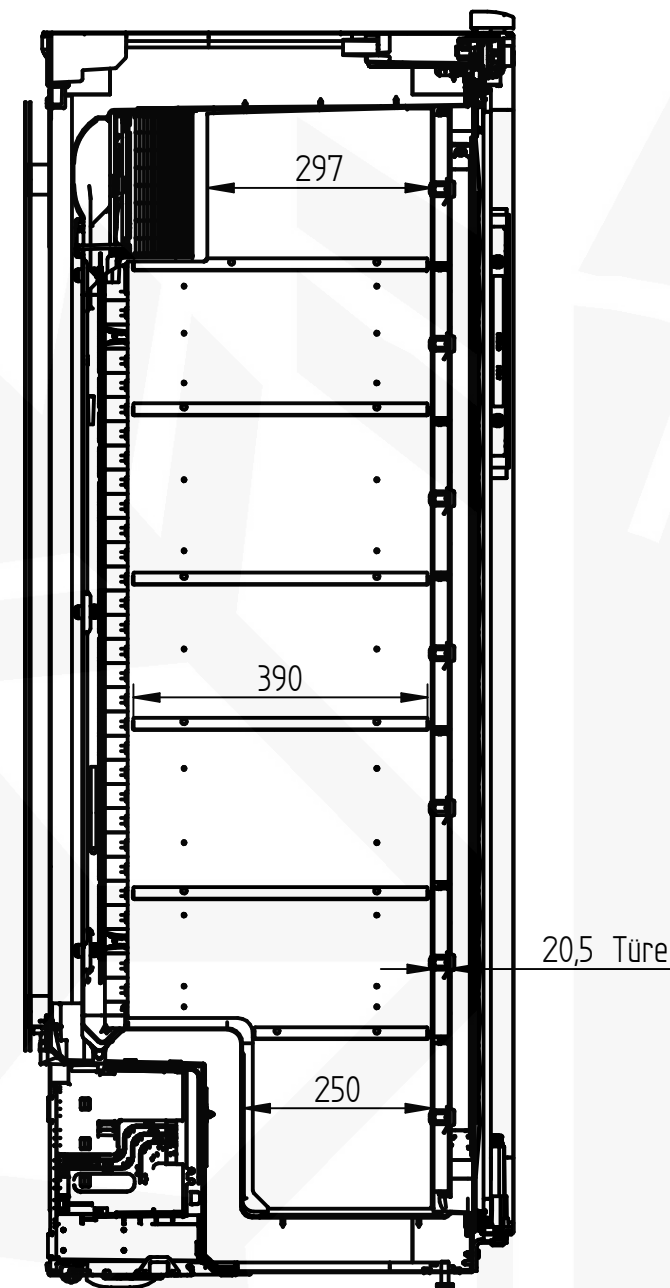
Schnitt A-A
