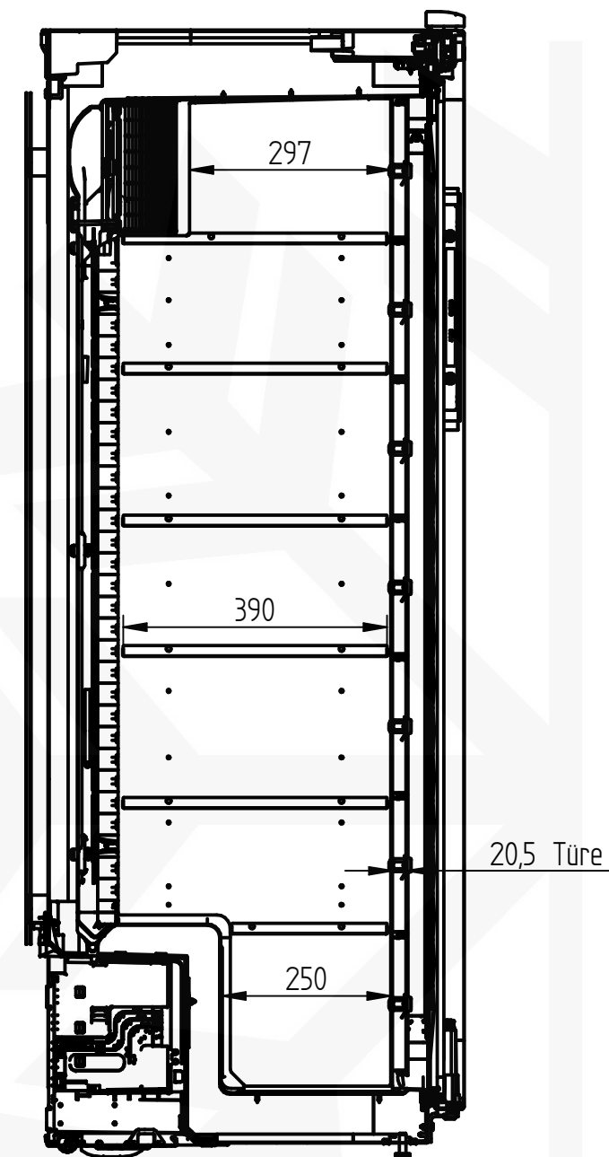
Schnitt A-A
