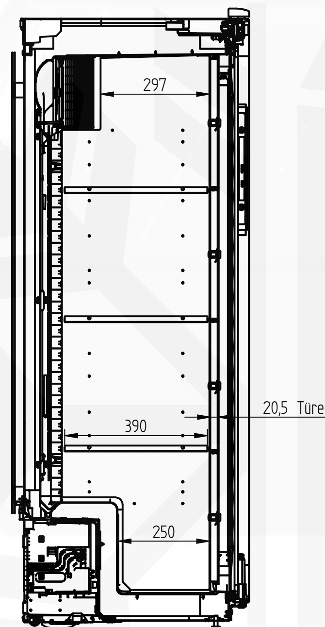
Schnitt A-A
