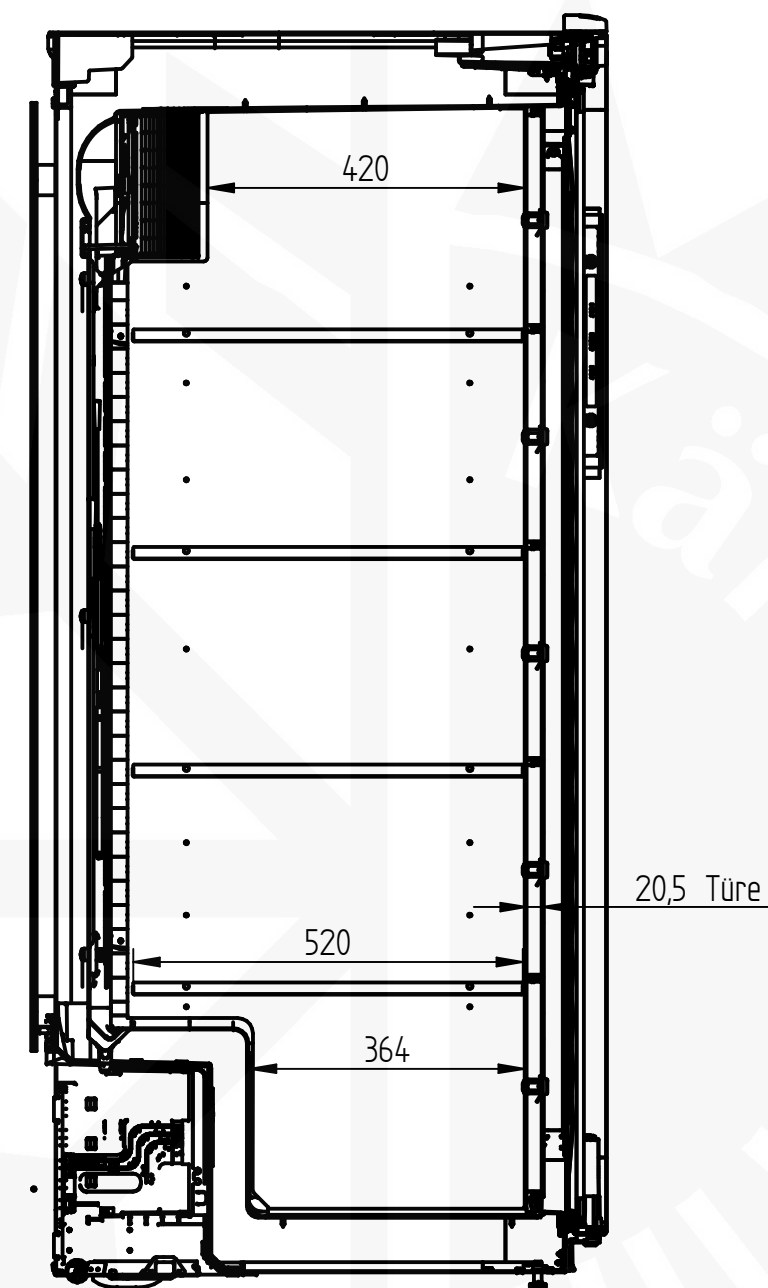
Schnitt A-A
