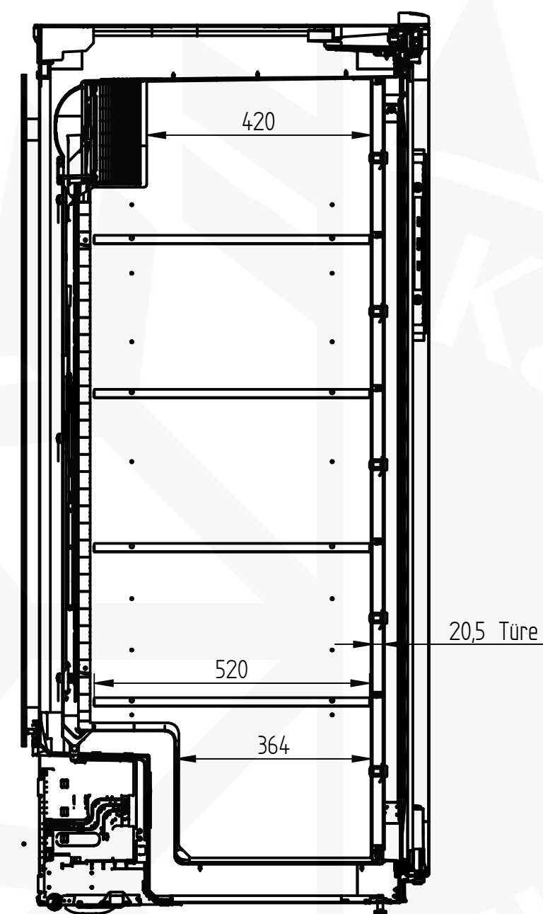
Schnitt A-A
