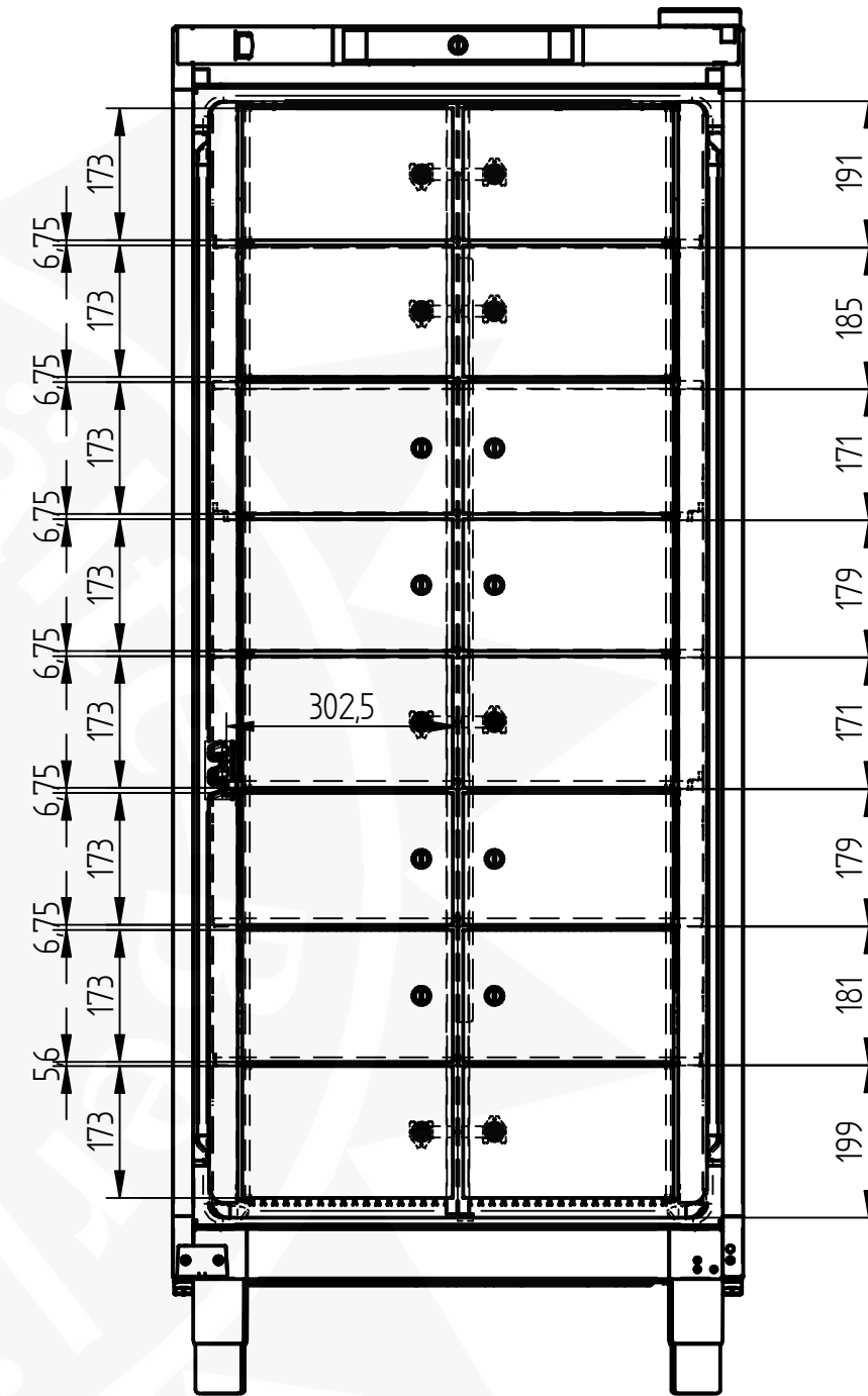
Ansicht ohne Tür
