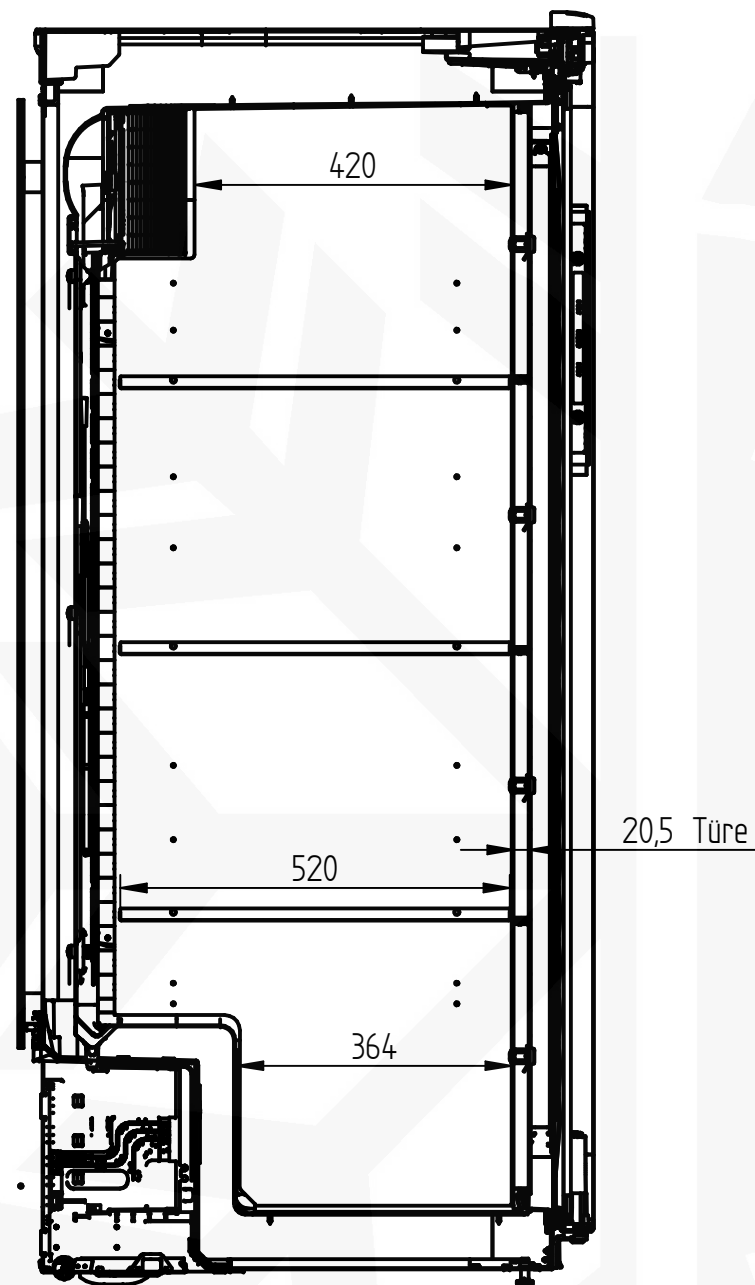
Schnitt A-A
