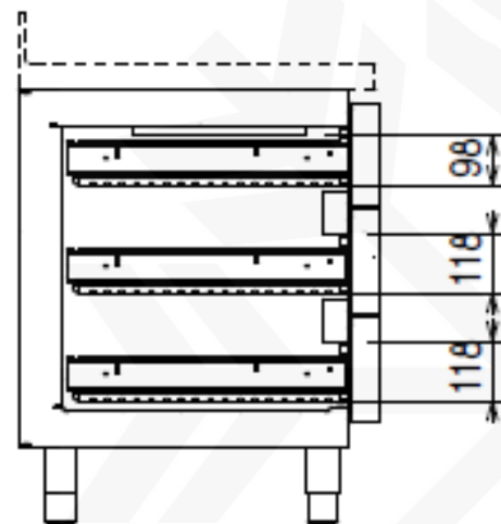
3x1/3 Schubladen
