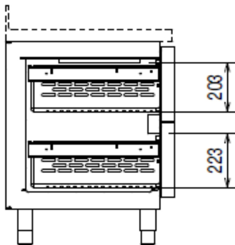
2x1/2 Schubladen
