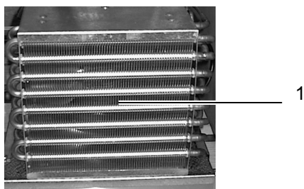
Abbildung 5-1 Kühlrippen am Verdampfer
