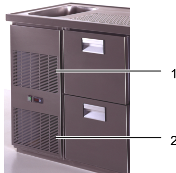
Abbildung 4-2: Lüftungsgitter des Kühlaggregats
