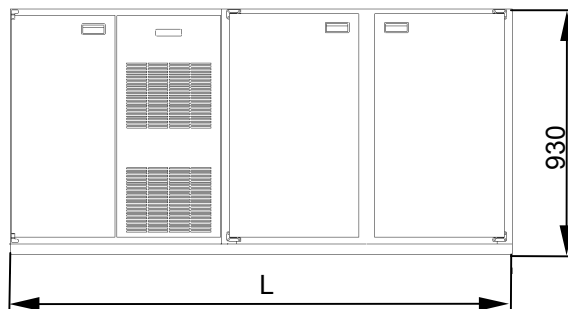
Abbildung 3-2: Abmaße Kühltheke
