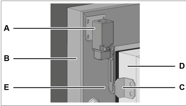
Stehender Einbau
