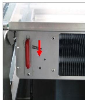
Abb. 6.18 Sichern: Beidseitig die roten Griffe nach unten schieben.
