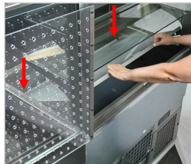
Abb. 6.16 Nach der Reinigung die Warenauslage beidseitig anheben und vorsichtig zurückschwenken. Darauf achten, dass die seitlichen Führungen der Warenauslage auf den Lagerbolzen aufliegen.
