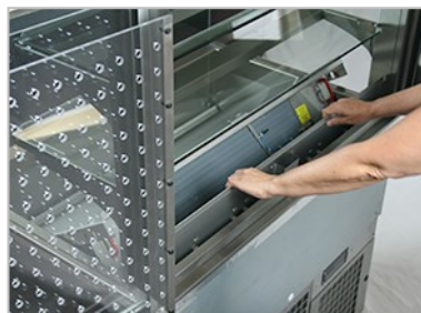
Abb. 6.6 Luftausblasblende entnehmen (bzw. einsetzen).
